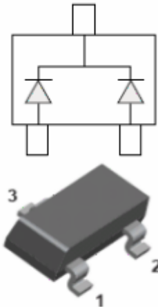
SOT-323
